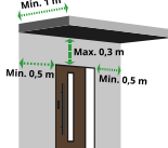
Zadaszenie drzwi
